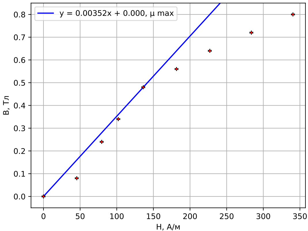
Зависимость В от H, Fe-Si
